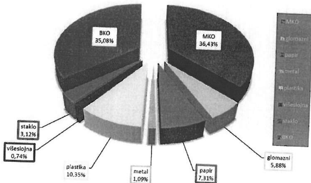
Grafikon 1 - Postotni udjeli pojedinih frakcija u komunalnom otpadu Općine Strahoninec
